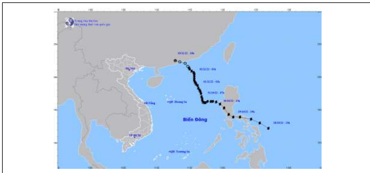
Hình 1. Bản đồ quỹ đạo bão số 7
