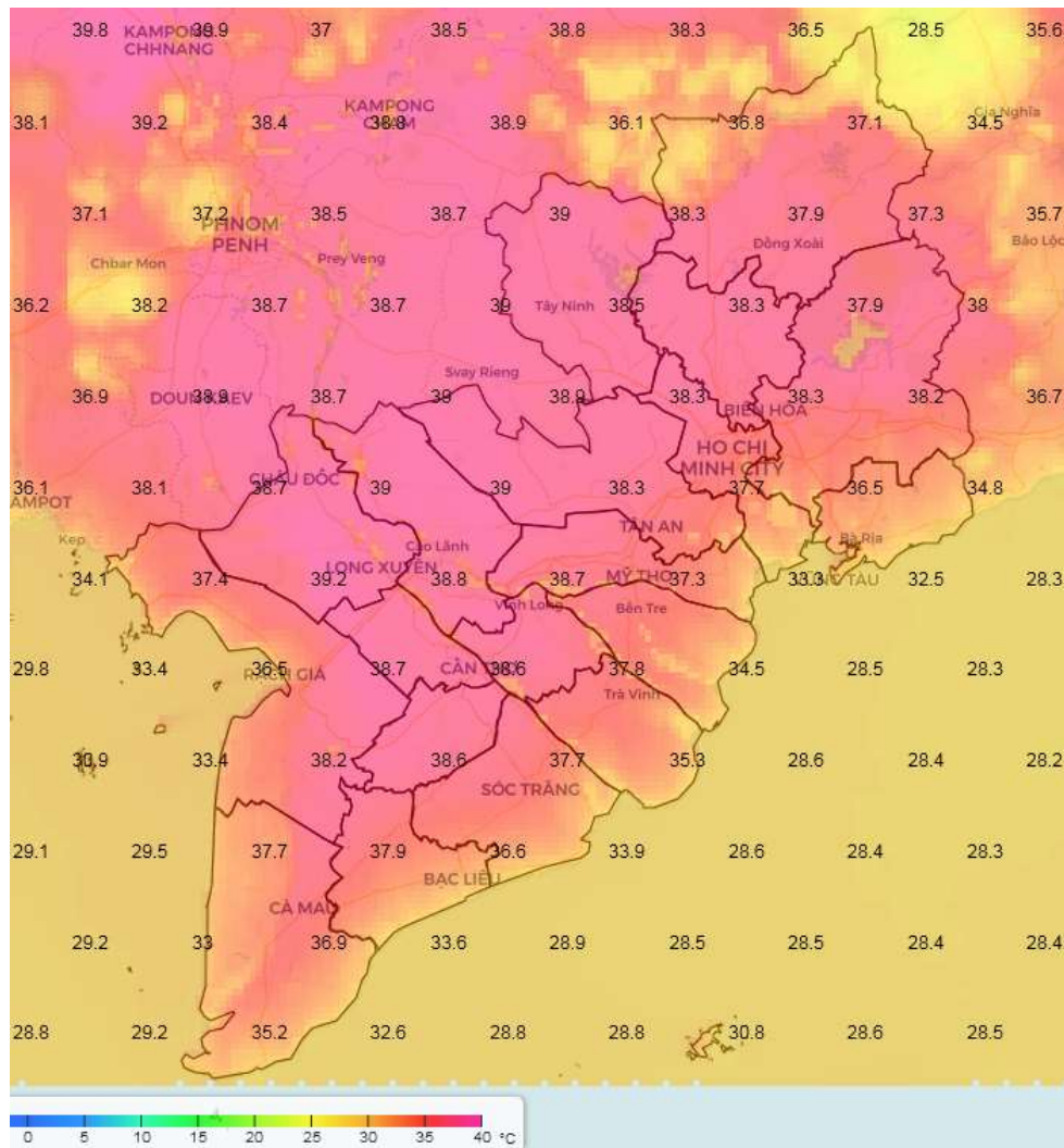
Bản đồ dự báo nhiệt độ cao nhất lúc 14h00 ngày 02-05-2024
