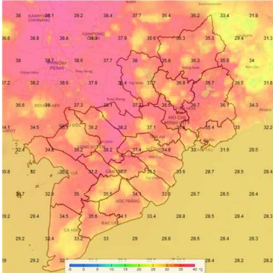
Bản đồ dự báo nhiệt độ cao nhất lúc 15h00 ngày 05-05-2024
