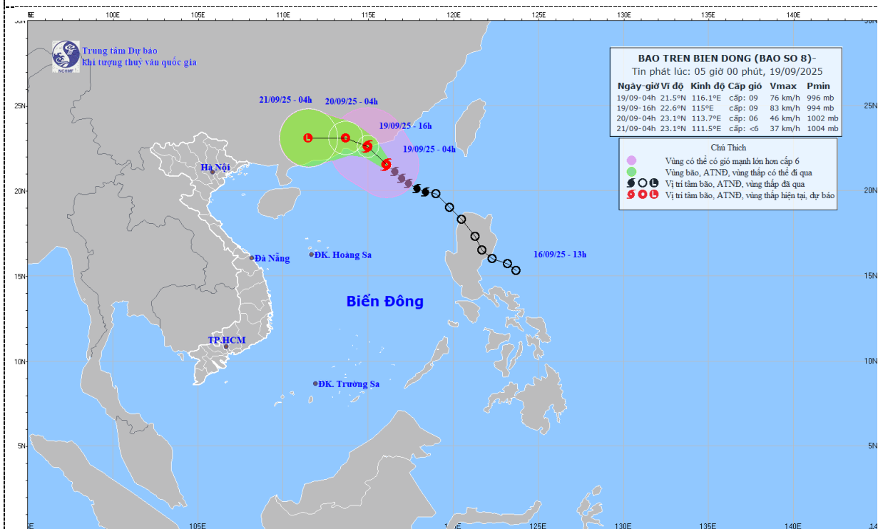
Hình 1. Bản đồ dự báo quỹ đạo và cường độ bão phát lúc 05h00 ngày 19/9/2025
