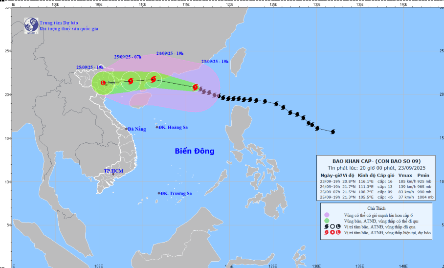
Hình 1. Bản đồ dự báo quỹ đạo và cường độ bão số 9 phát lúc 20h00 ngày 23/9/2025
