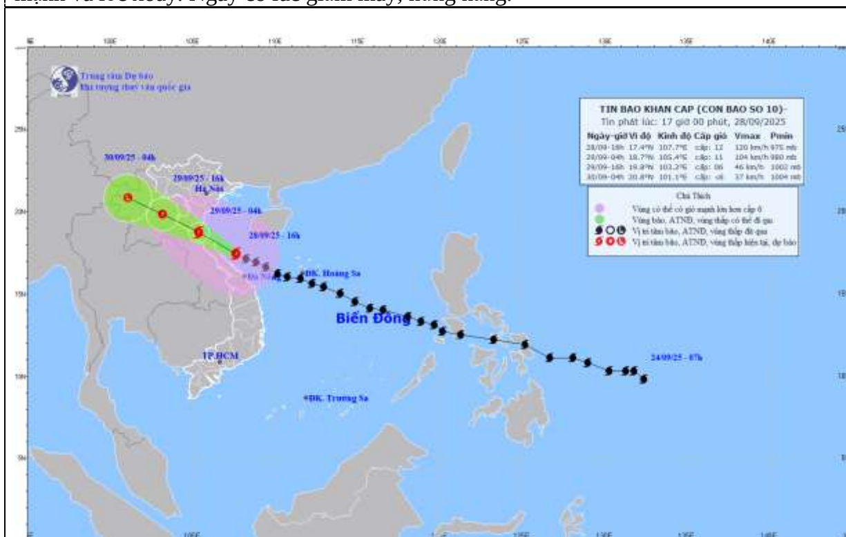
Hình1. Bản đồ dự báo quỹ đạo và cường độ bão số 10 phát lúc 17h00 ngày 28/9/2025
