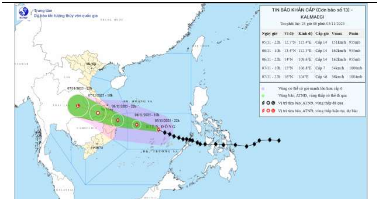
Hình 1. Bản đồ dự báo quỹ đạo và cường độ bão số 13 (Kalmaegi) phát lúc 23h00 ngày 05/11/2025. Bản tin tiếp theo được phát lúc 02h00 ngày 06/11.
