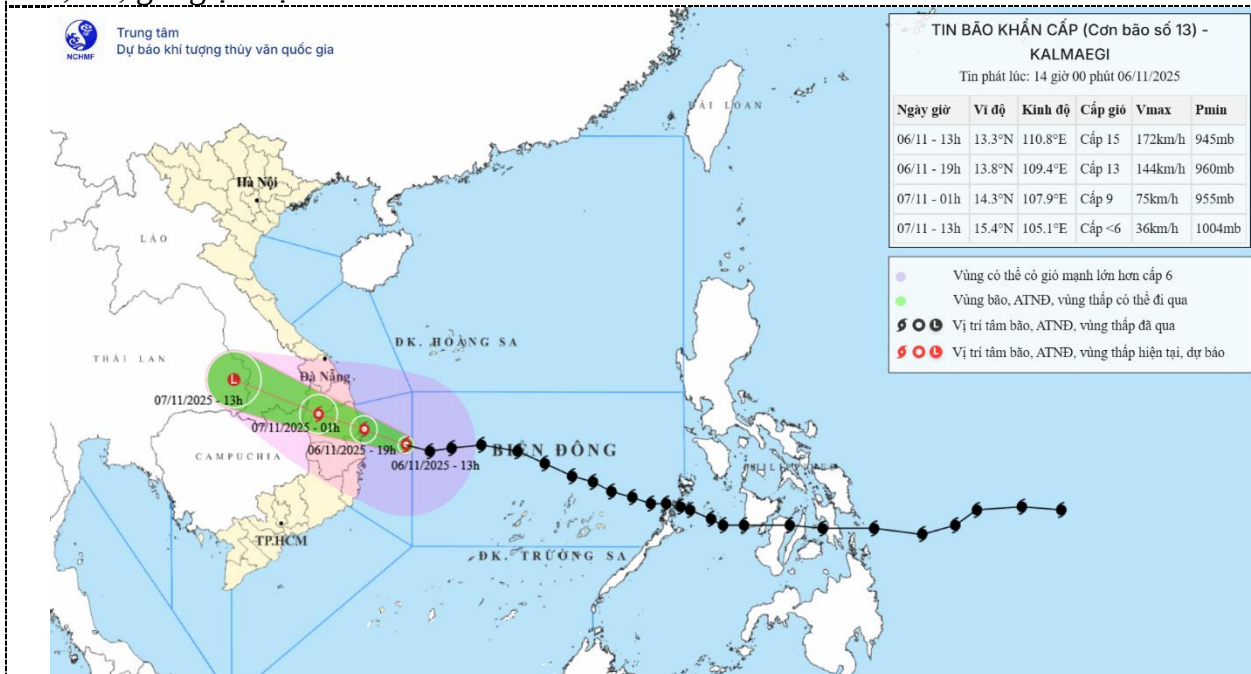
Hình 1. Bản đồ dự báo quỹ đạo và cường độ bão số 13 (Kalmaegi) phát lúc 14h00 ngày 06/11/2025
